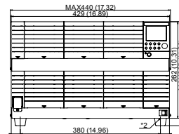
429(16.89)W×262(10.31)H×520(20.47)Dmm(inches)
